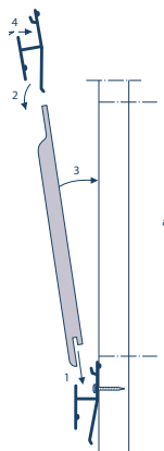
instalación fija
