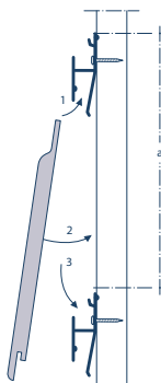
instalación desmontable (posibilidad de colocación asegurada)
