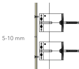
Estructura de soporte en aluminio con junta horizontal abierta
