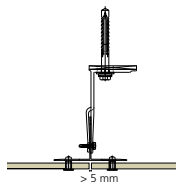
Estructura de aluminio, solución a la altura de las juntas verticales
