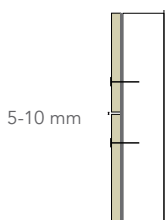
Estructura de soporte en madera con junta horizontal abierta
