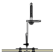
Estructura de aluminio, solución a la altura de las juntas verticales
