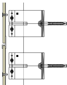
Estructura de aluminio con junta horizontal cerrada
