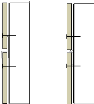
Estructura de madera con junta horizontal cerrada (a la izquierda) y semicerrada (a la derecha)
