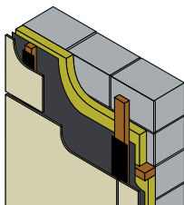
Estructura de madera
